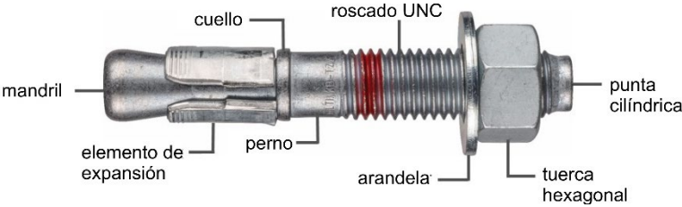
FIGURA 1—HILTI KWIK BOLT TZ (KB-TZ2) DE ACERO AL CARBONO
