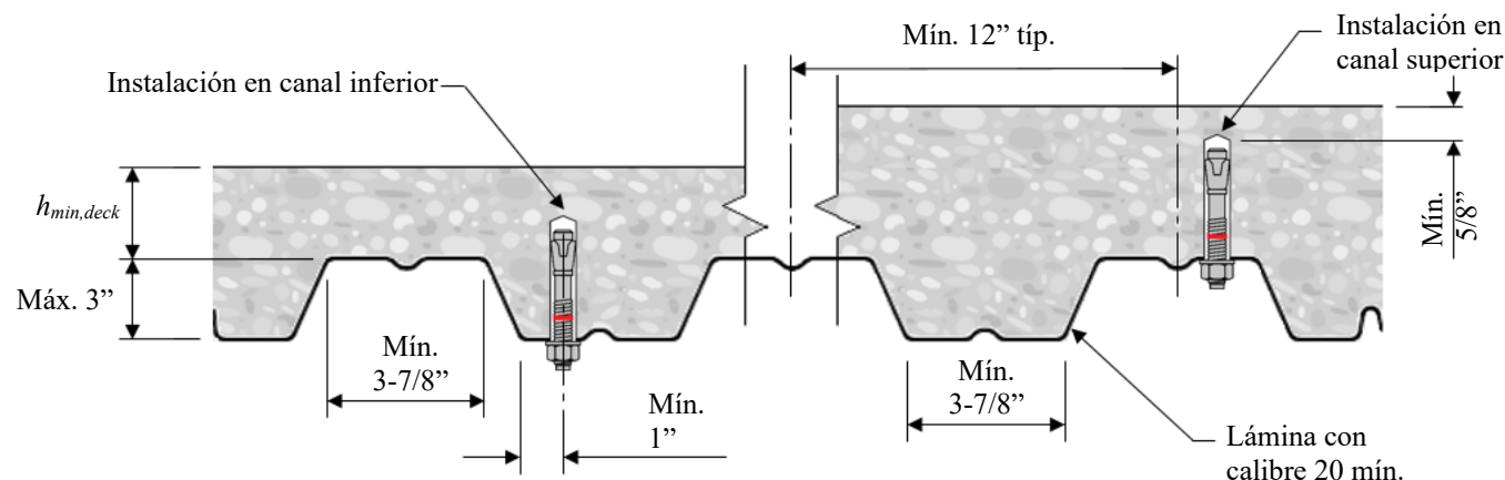
FIGURA 5A—KB-TZ2 EN EL ELEMENTO DE CONCRETO RELLENO EN LOSAS COMPUESTAS – LÁMINA W
